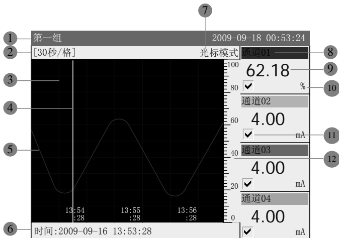
横向历史曲线
