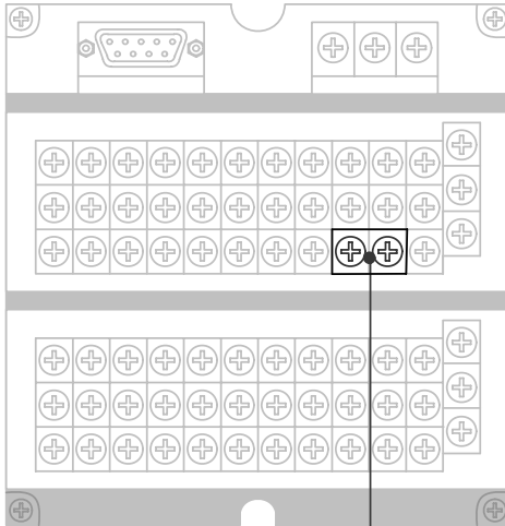
外部开关输入端子
