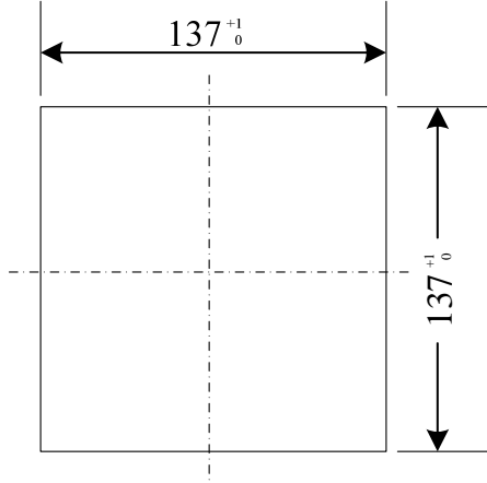
集装表开孔尺寸
