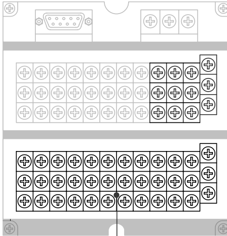
输入输出端子
