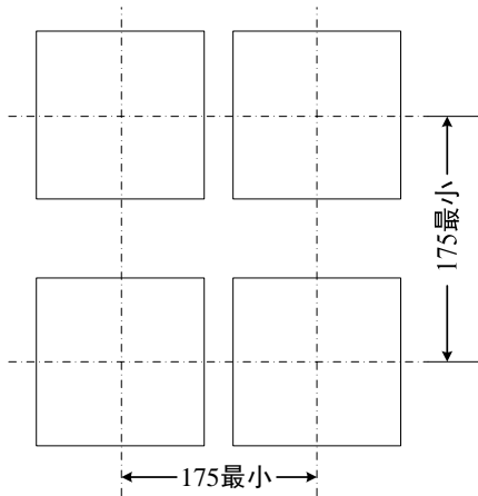
集装表开孔尺寸
