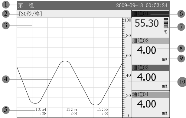
实时曲线显示举例（横向）
